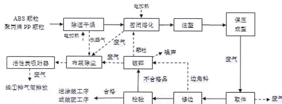
图 2.3-2 注塑工艺流程及产污节点图
