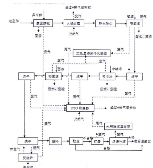
图 2.3-3 涂装工艺流程及产污节点图
