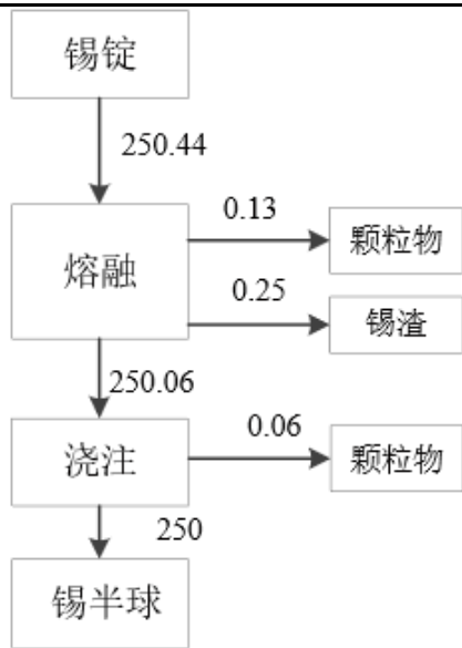
图 2-4 锡半球物料平衡图（单位 t/a）
