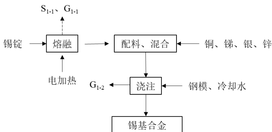
图 2-6 锡基合金工艺流程与产排污环节
