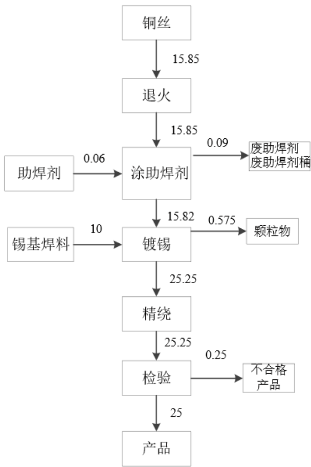
图 2-5 光伏焊带物料平衡图（单位 t/a）
