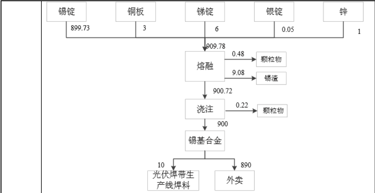
图 2-2 锡基合金物料平衡图 (单位 t/a)
