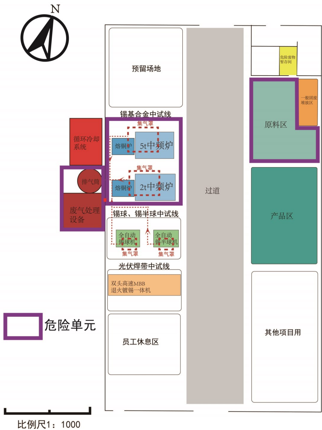
图 3-1 危险单元分布图
