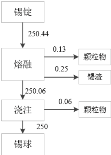
图 2-2 锡基合金物料平衡图 (单位 t/a)
