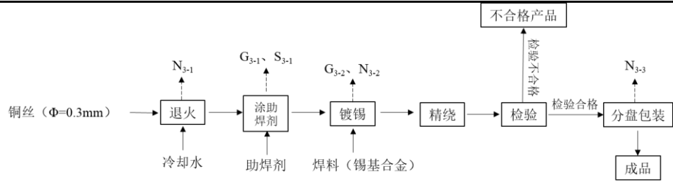
图 2-8 光伏焊带中试生产工艺流程与产污环节
