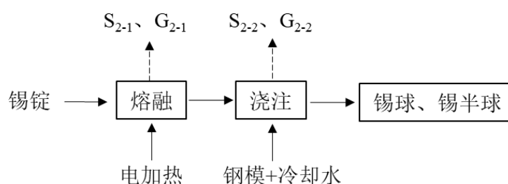
图 2-7 锡球、锡半球工艺流程与产排污环节
